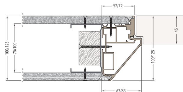
Marco en pared de una placa de yeso - Grosor pared acabada 100/125/150 mm
