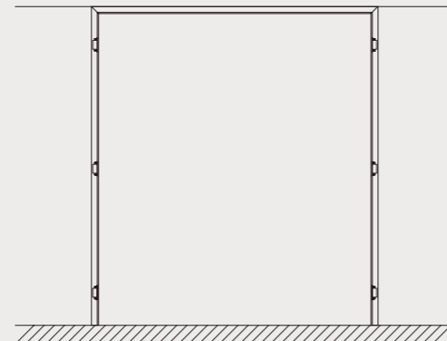
marco abatible hoja doble con travesaño a ras de techo
