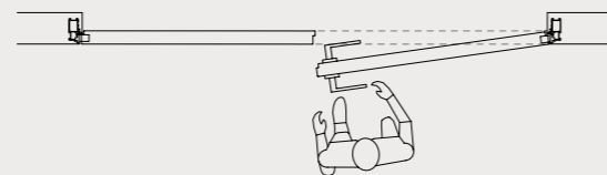
puerta derecha tirar - puerta izquierda fija
