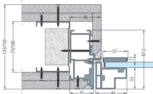
Contramarco en la pared de cartón yeso con tres placas - Espesor pared acabada 125/150 mm
